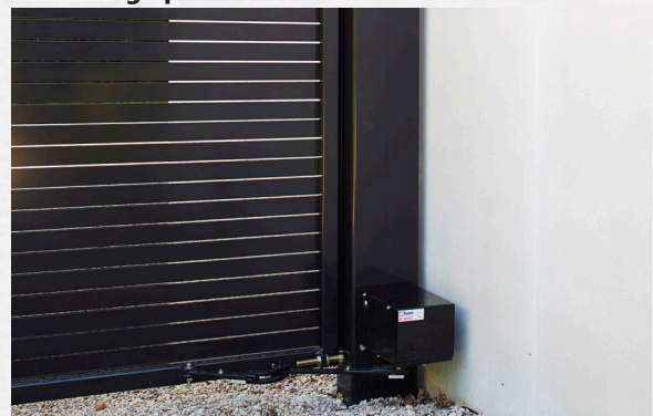
Vleugelpoort met MCH150-motor binnenaanzicht
